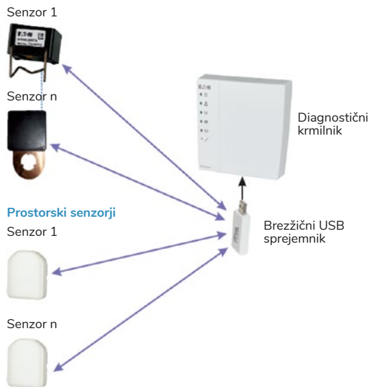
Slika 2: Konfiguracija merilnih senzorjev
