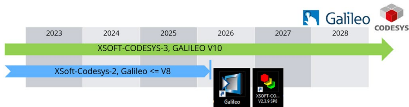
Slika 5: Programska oprema
